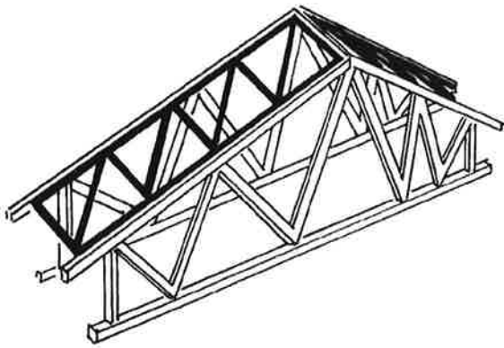
Kuva 16. Katon jäykistämiseen käytettävät NR-vaakaristikot.
