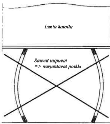
Kuva 13. NR-rakenne ei kestä suunniteltua kuormaa, jos sisäsauvojen nurjahdustuet jäävät asentamatta.
